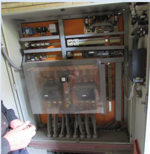
شکل ۲- تابلو برق غیراستاندارد مربوط به روشنایی سالن مطالعه، تابلو برق استاندارد دیزل ژنراتور
